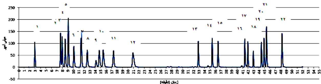
شکل ۴: کروماتوگرام مربوط به اسیدآمین‌های آزاد موجود در گرده زنبورعسل هیدرولیز شده با آنزیم آلکالاز شامل: ۱. گلوتامات، ۲. سرین، ۳. آسپارازین، ۴. گلابسین، ۵. گلوتامین، ۶. بتا-آلانین، ۷. تائورین، ۸. هیستیدین، ۹. ترئونین، ۱۰. آلانین، ۱۱. آرژنین، ۱۲. پرولین، ۱۳. تیروزین، ۱۴. والین، ۱۵. متیونین، ۱۶. ایزولوسین، ۱۷. لوسین، ۱۸. نورولوسین (استاندارد داخلی)، ۱۹. فنیل‌آلانین، ۲۰. تربیتوفان، ۲۱. اورنیتین، ۲۲. لیزین
